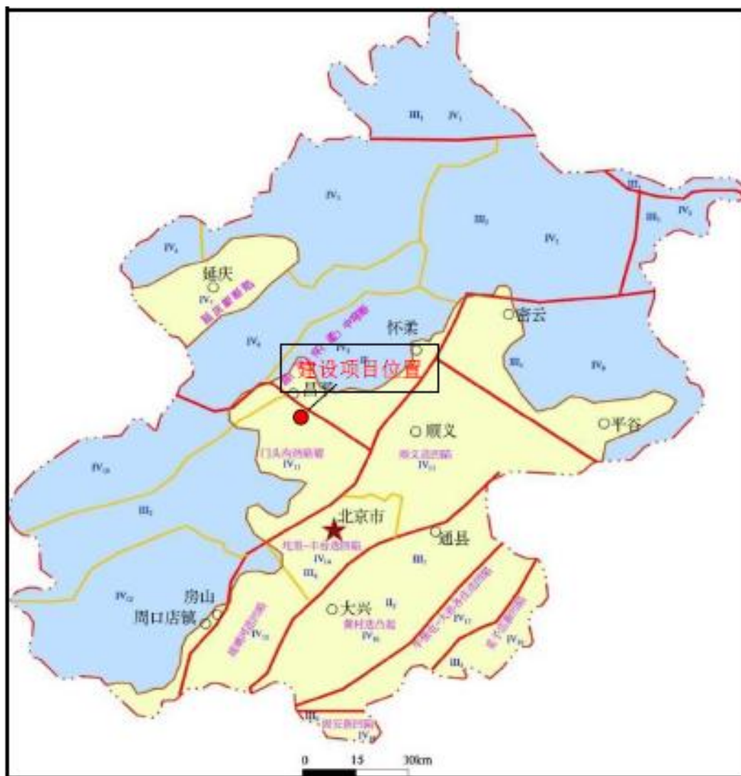
图 4.1-1 北京市地质构造单元划分图
