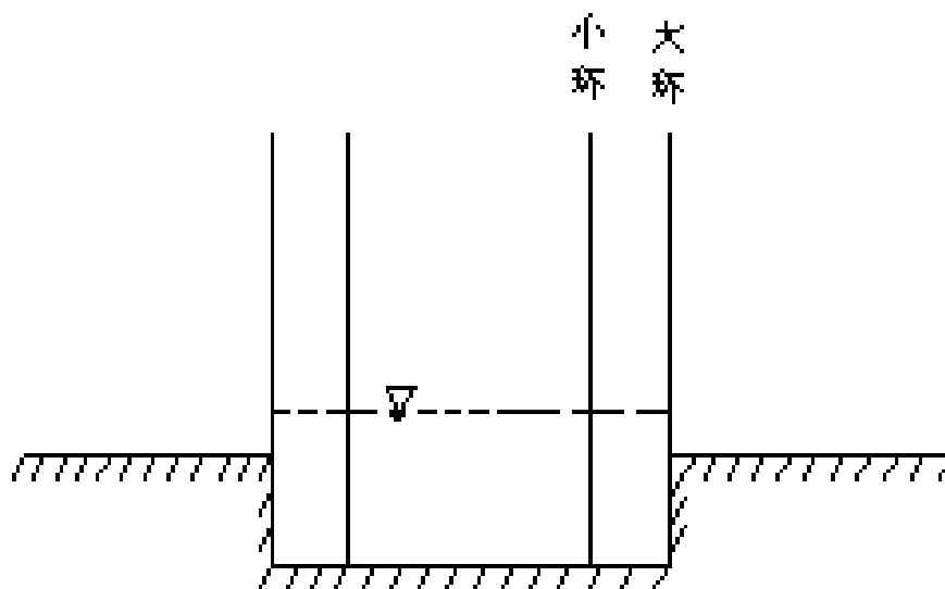
图 4.2-6 双环渗水试验装置示意图
