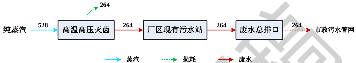
图 3.6-2 本项目蒸汽平衡情况一览表 ( \text{m}^3/\text{a} )
