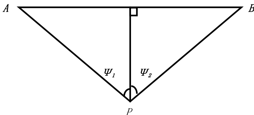
图 5-4 有限路段的修正函数 (A—B 为路段，P 为预测点)
