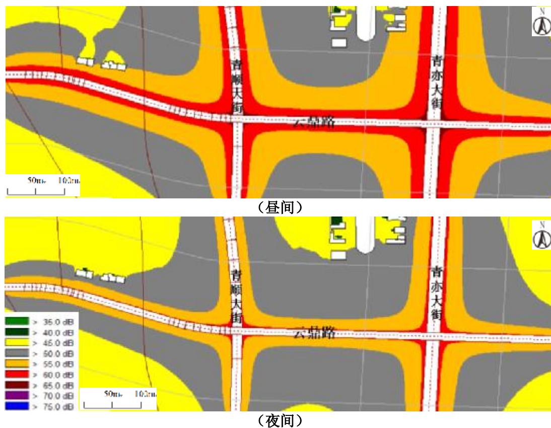
图 5-5 运营远期噪声预测结果二维图
