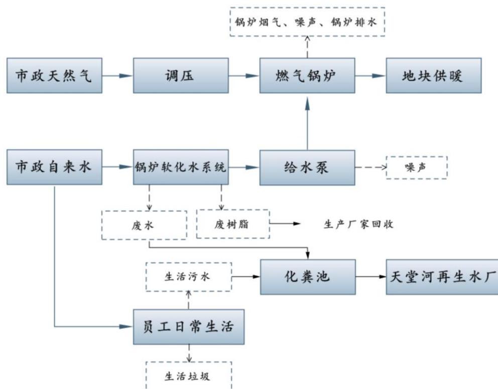
图4 生产工艺流程及产污环节示意图
