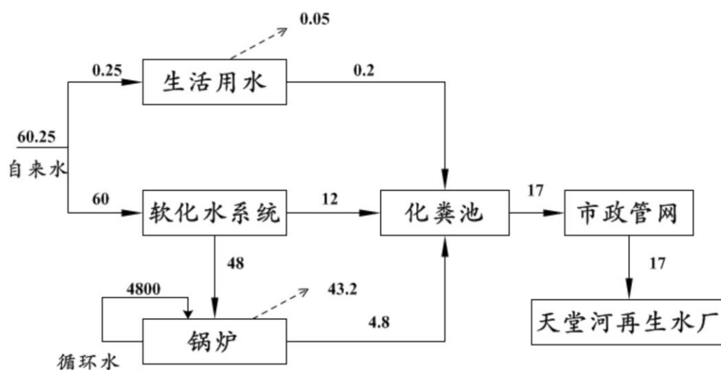
图3 本项目水平衡图 单位：m 3 /d
