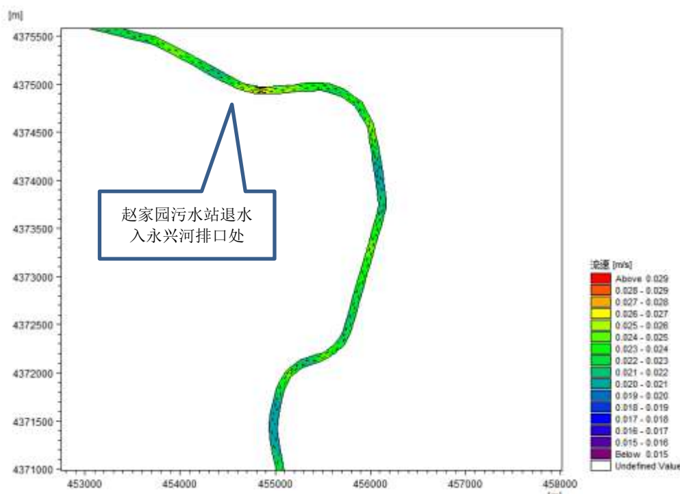
图 4.1-5 流速分布图
