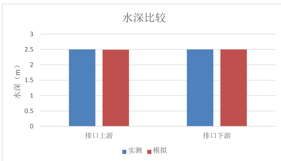
图 4.1-4 流速验证结果对比图
