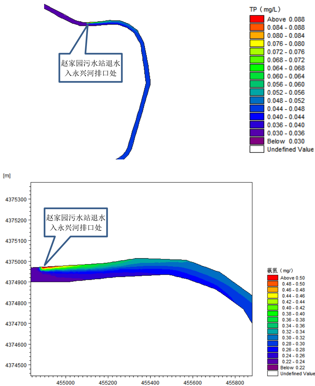
图 4.1-10 非正常排放工况下永兴河氨氮浓度变化图
