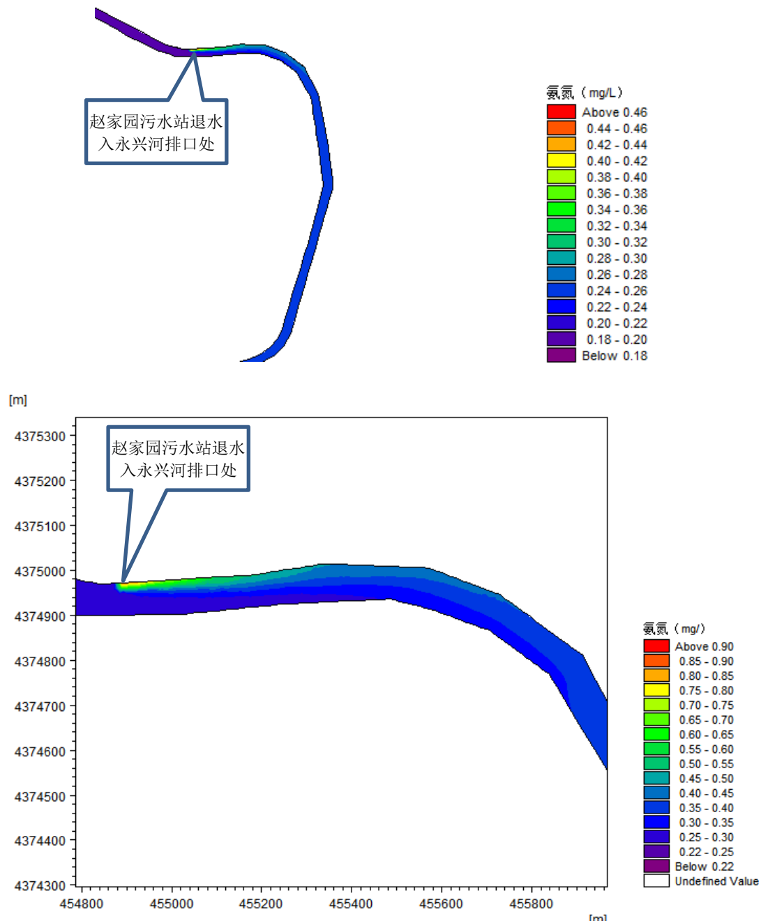
图 4.1-13 事故排放工况下永兴河氨氮浓度变化图
