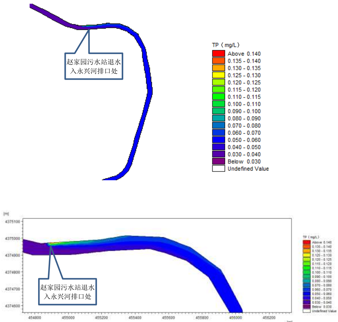
图 4.1-14 事故排放工况下永兴河 TP 浓度变化图
