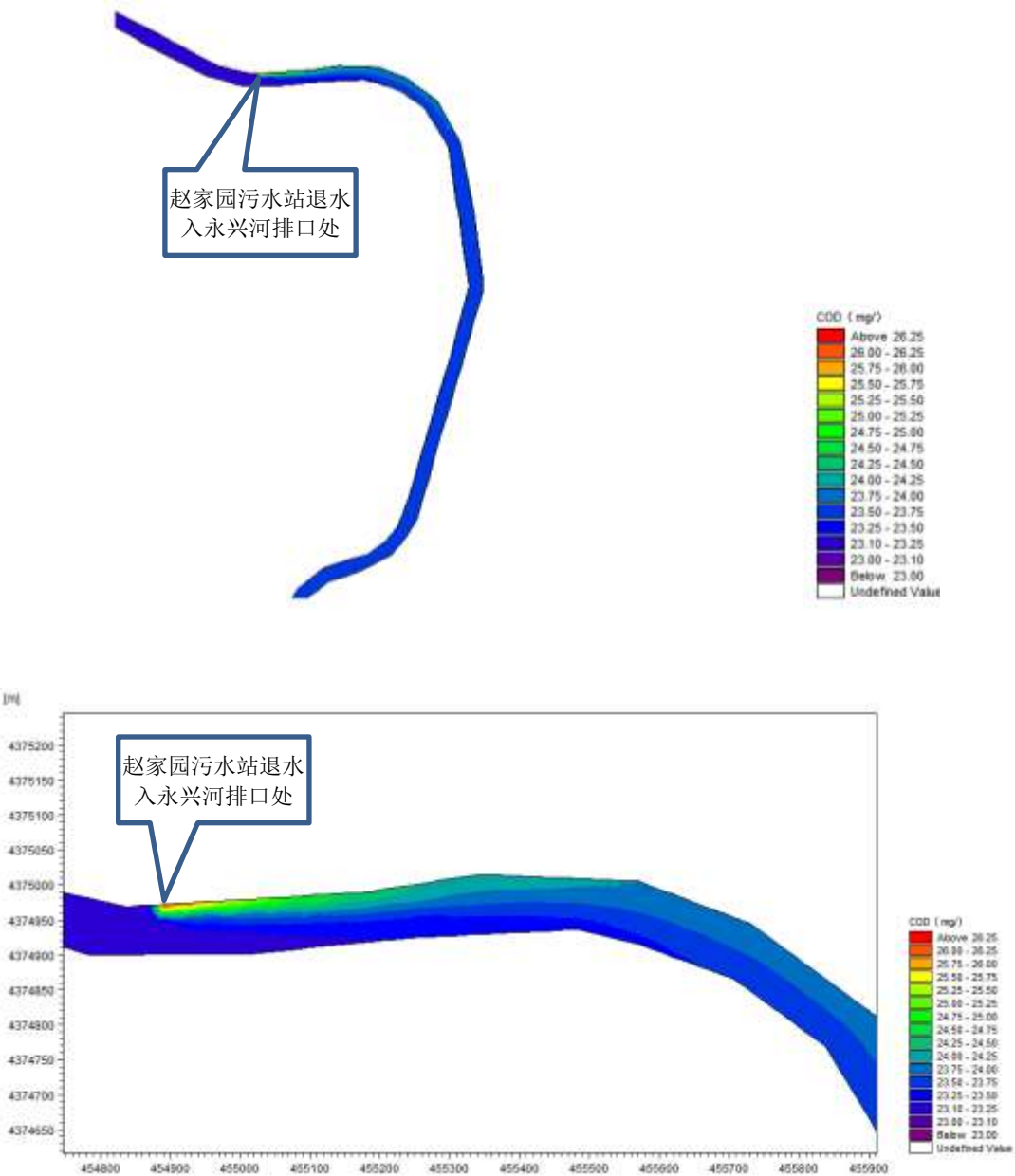
图 4.1-9 非正常排放工况下永兴河 COD Cr 浓度变化图
