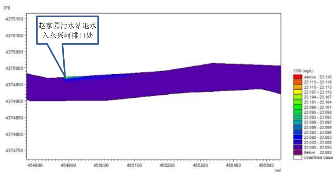
图 4.1-6 正常排放工况下永兴河 COD Cr 浓度变化图
