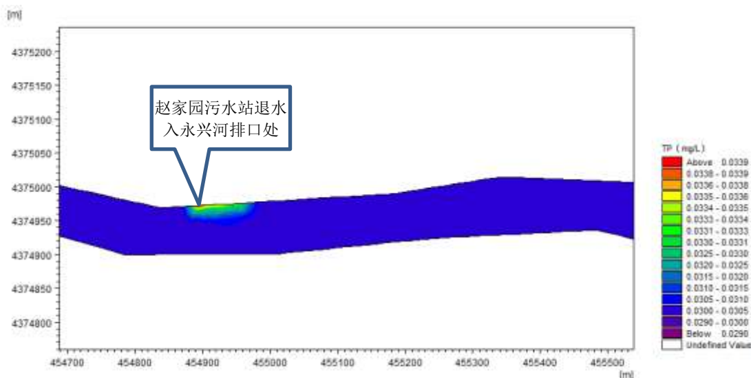
图 4.1-8 正常排放工况下永兴河 TP 浓度变化图
