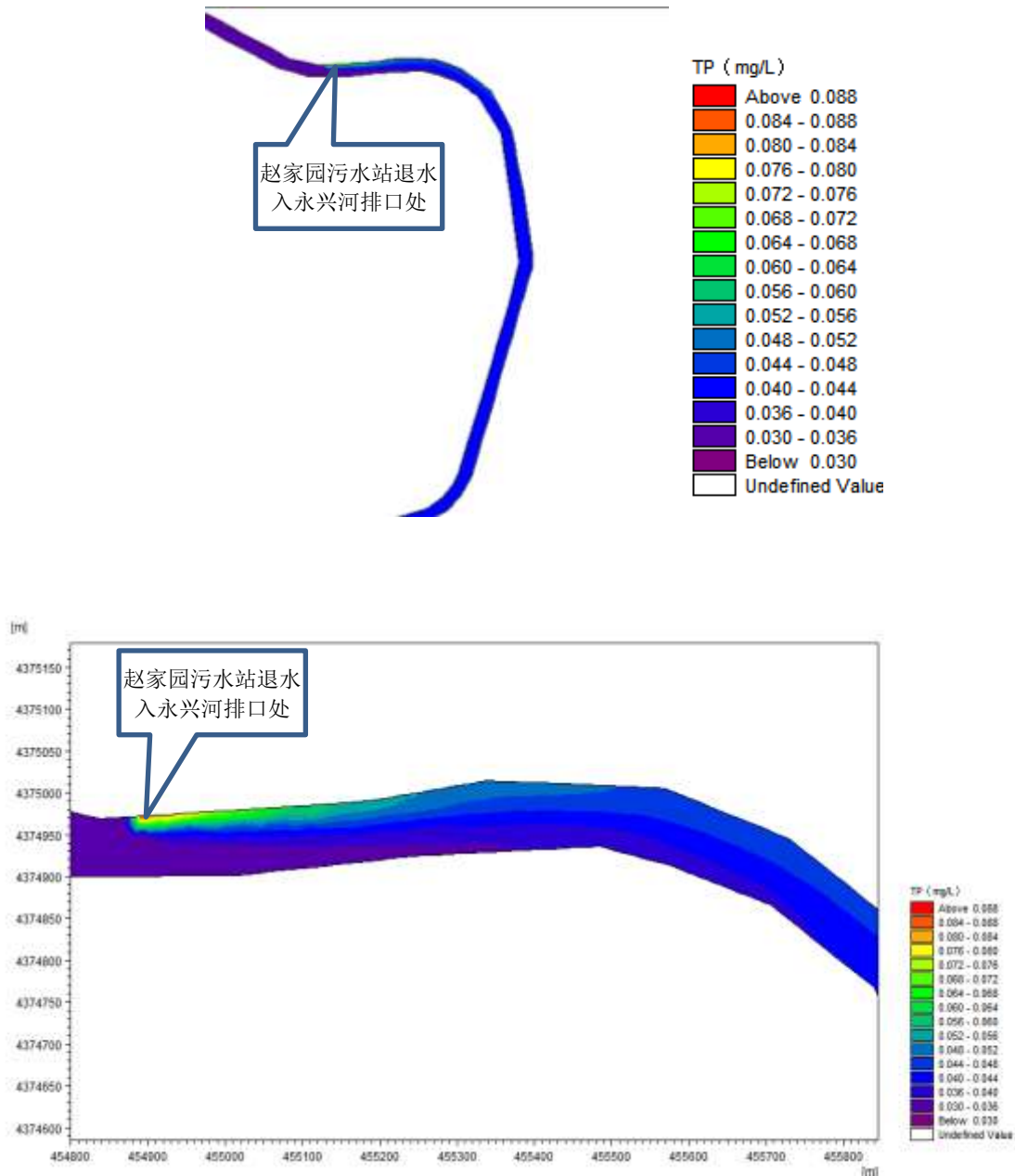
图 4.1-11 非正常排放工况下永兴河 TP 浓度变化图
