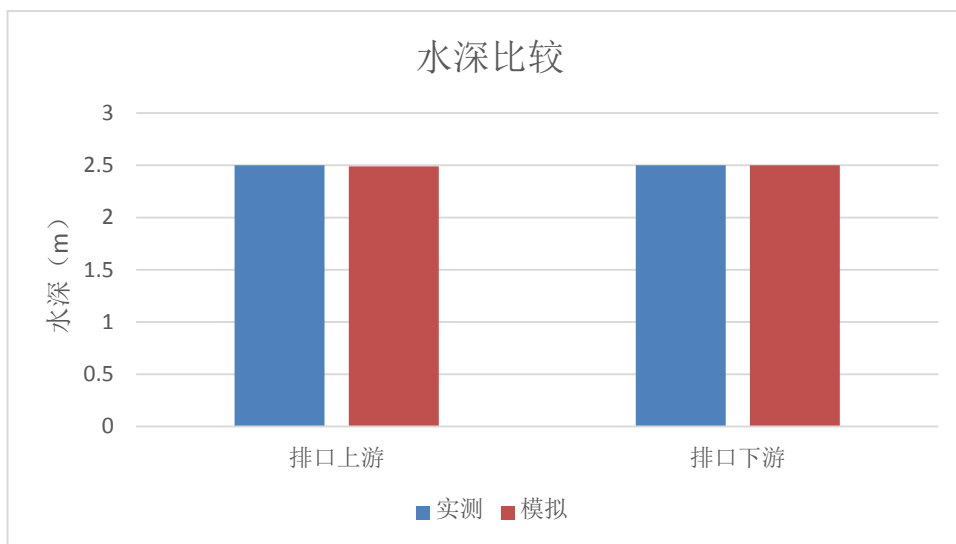
图 4.1-3 水深验证结果对比图
