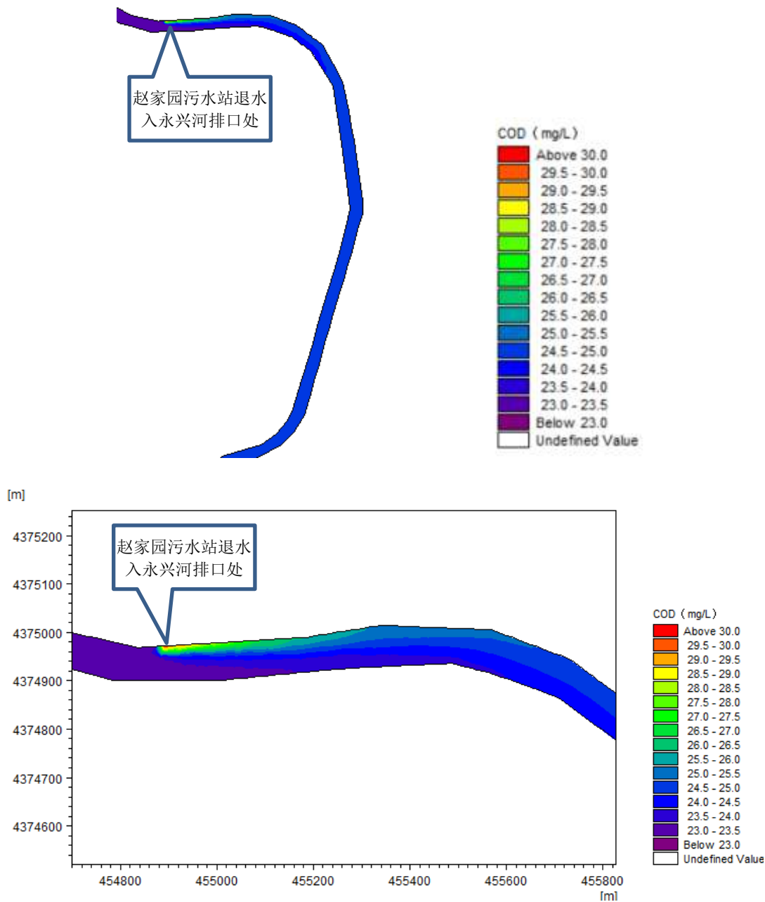
图 4.1-12 事故排放工况下永兴河 \text{COD}_{\text{Cr}} 浓度变化图
