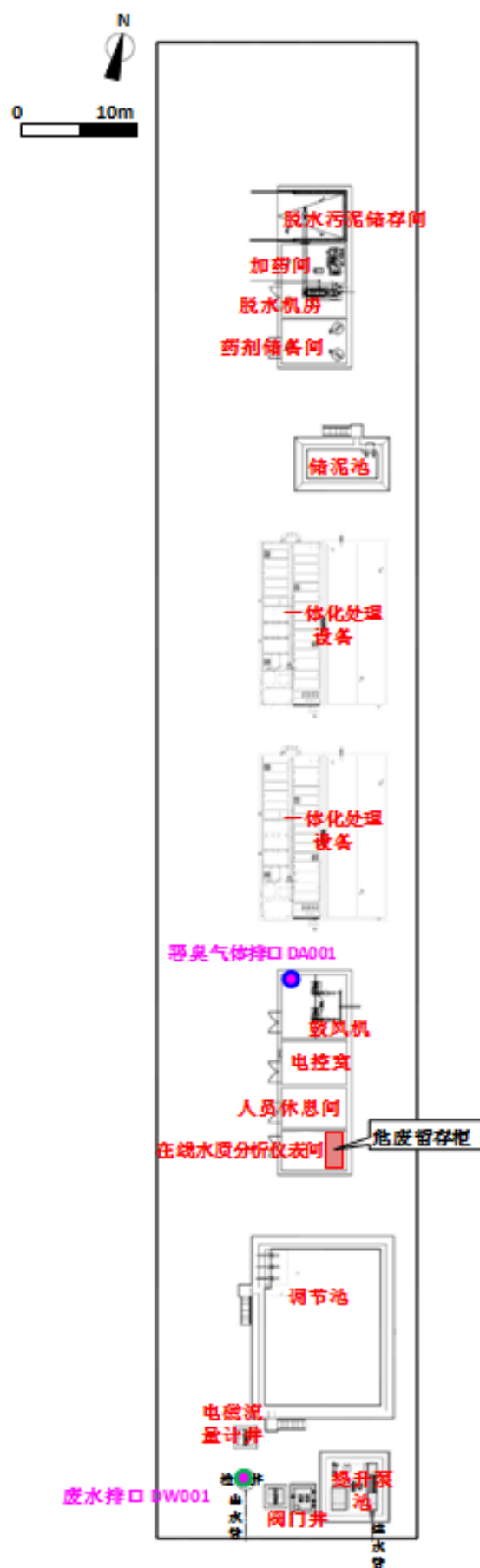
附图 2 厂区总平面布置图
