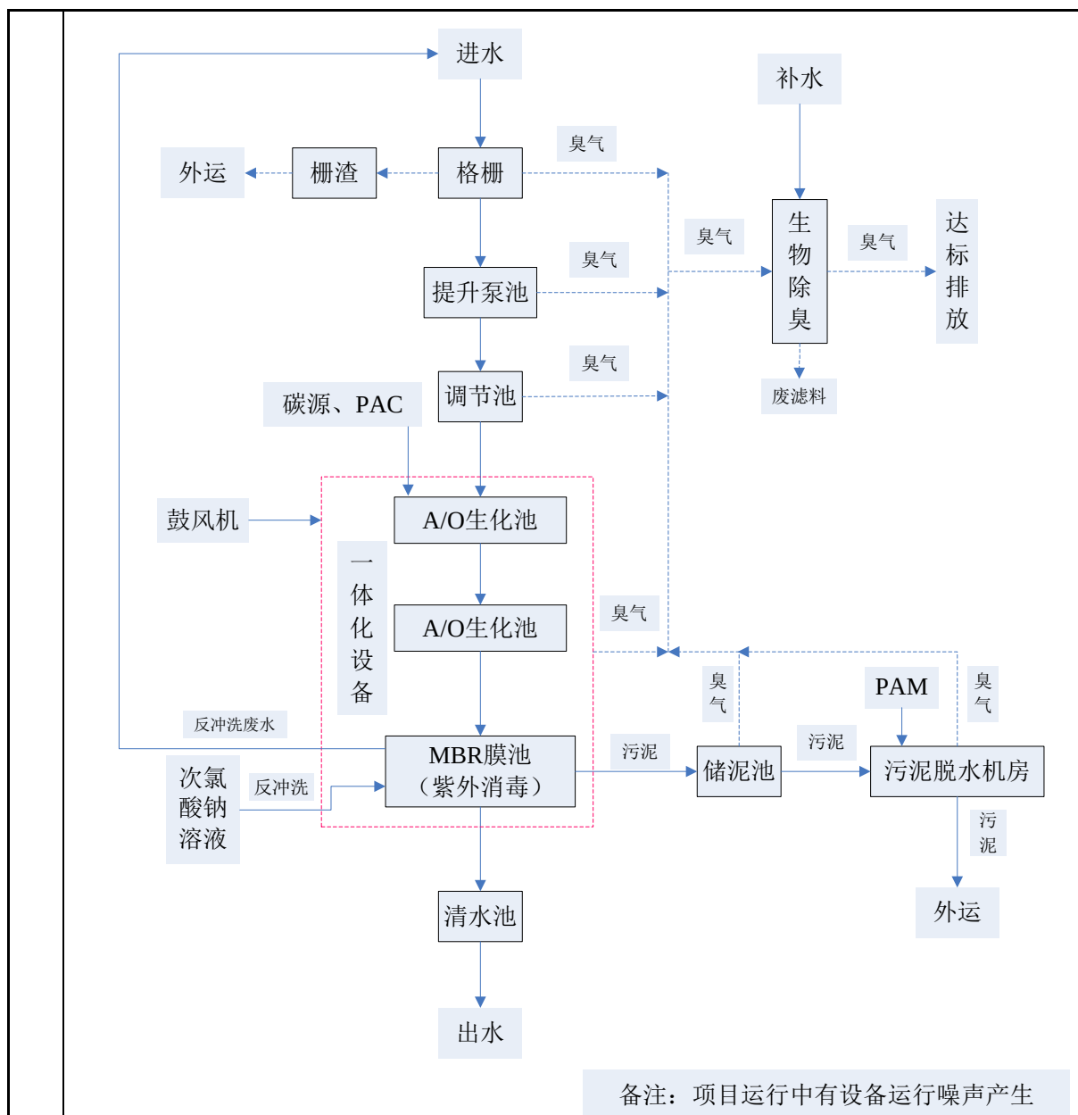
图2-2 生产工艺流程及产污环节示意图
