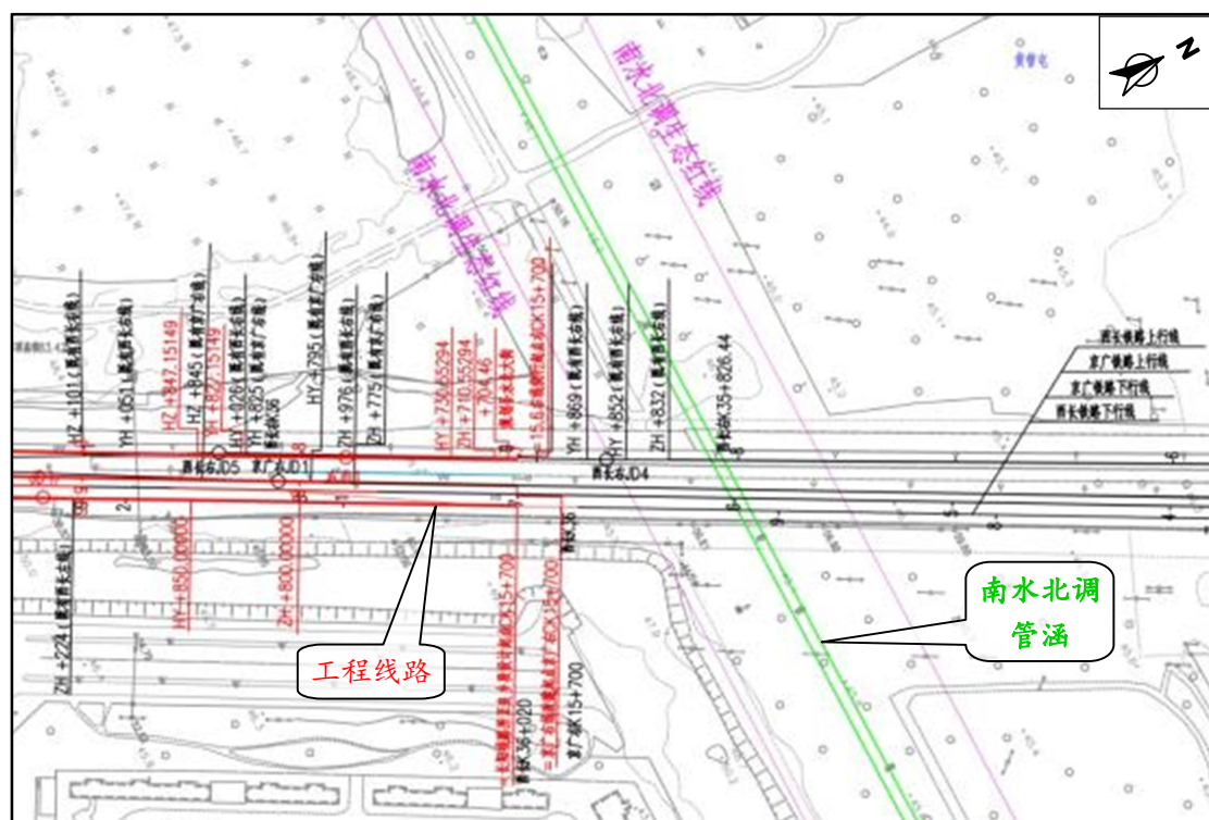
图 7.2-1 工程线路与南水北调管涵位置关系图
