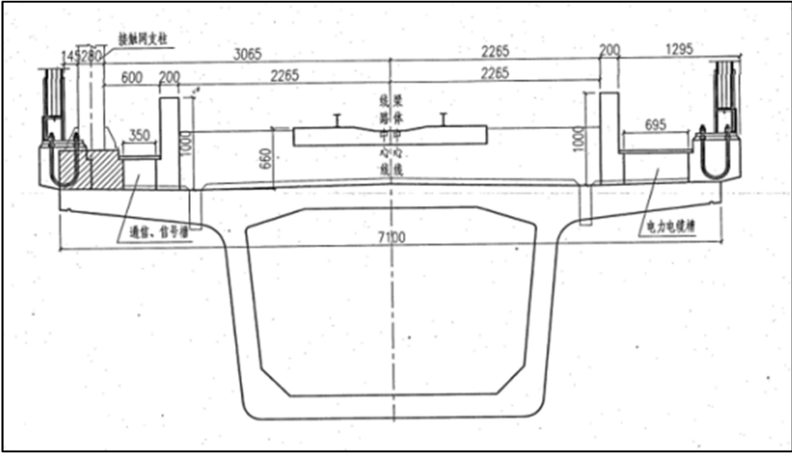
图 2.2-4 桥梁标准断面图
