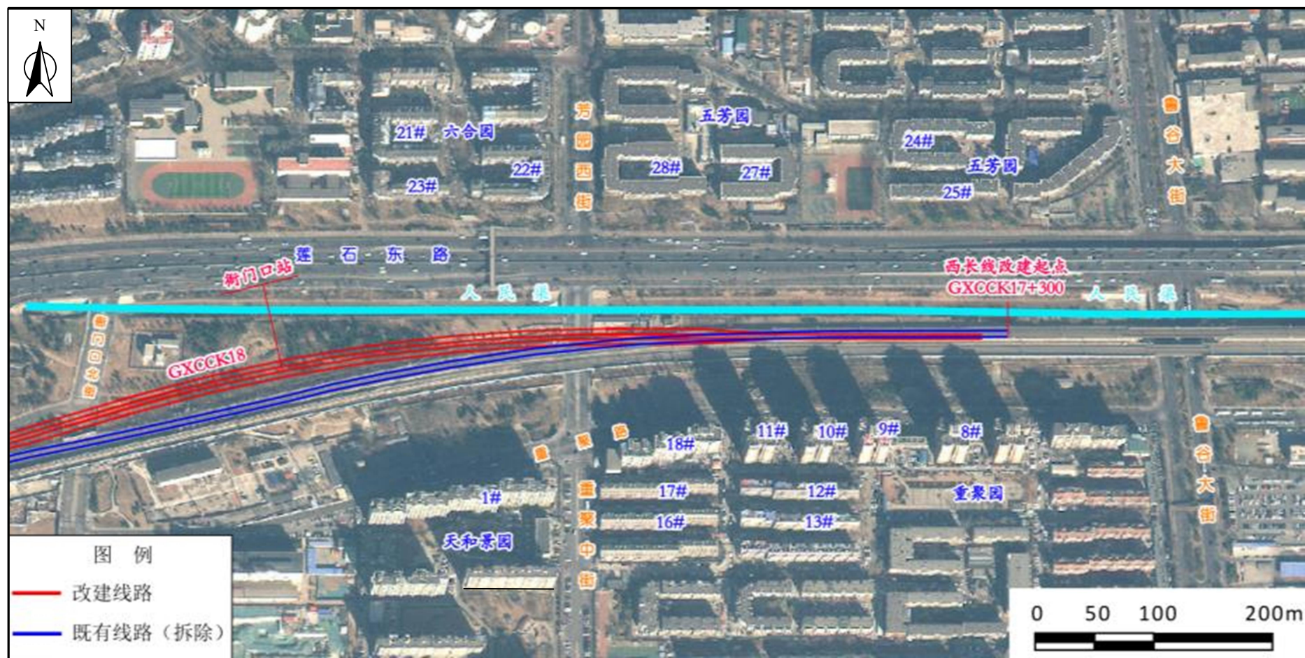
图 1.5-2 环境保护目标位置示意图（衙门口站）
