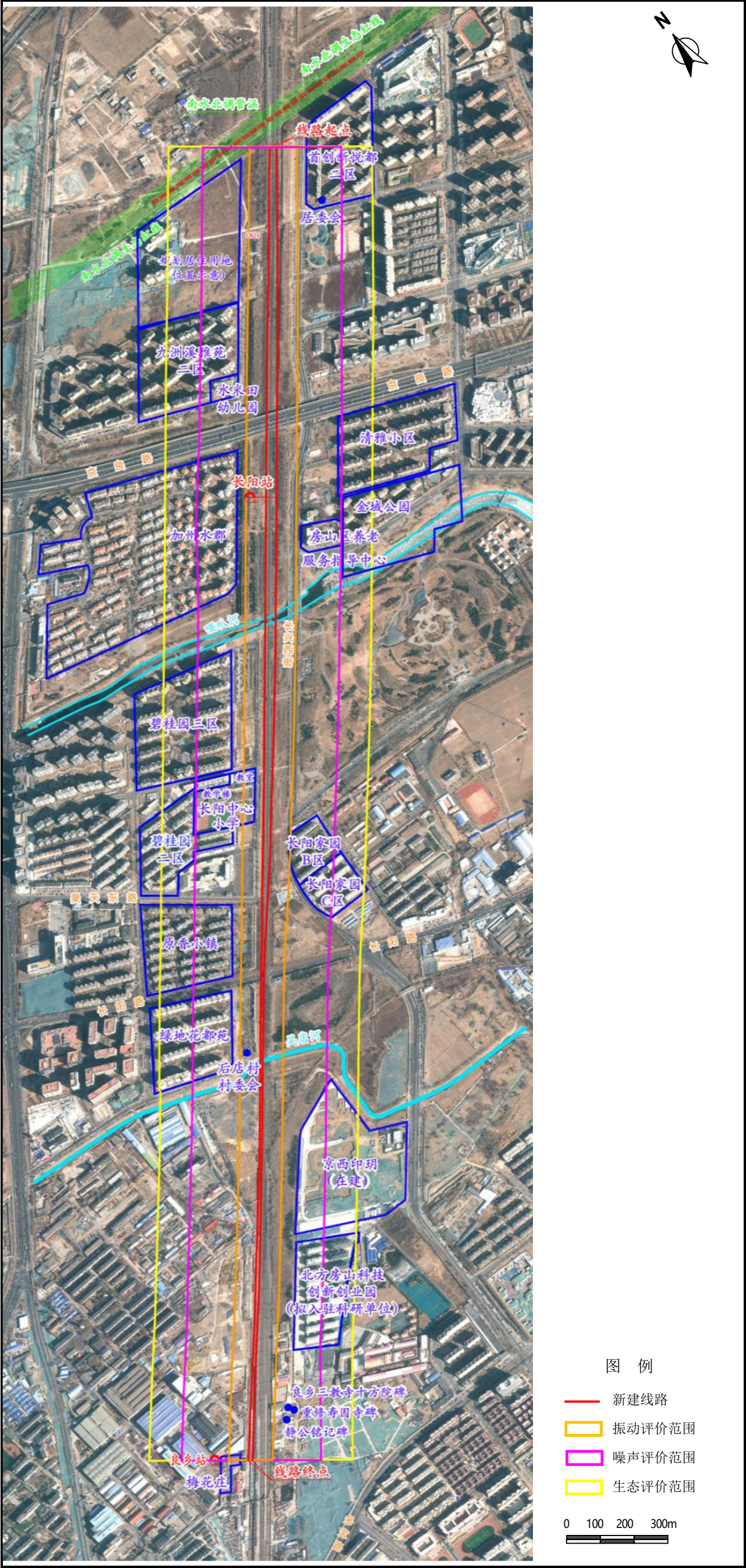
图 1.4-3 长阳村线路所至良乡段评价范围图
