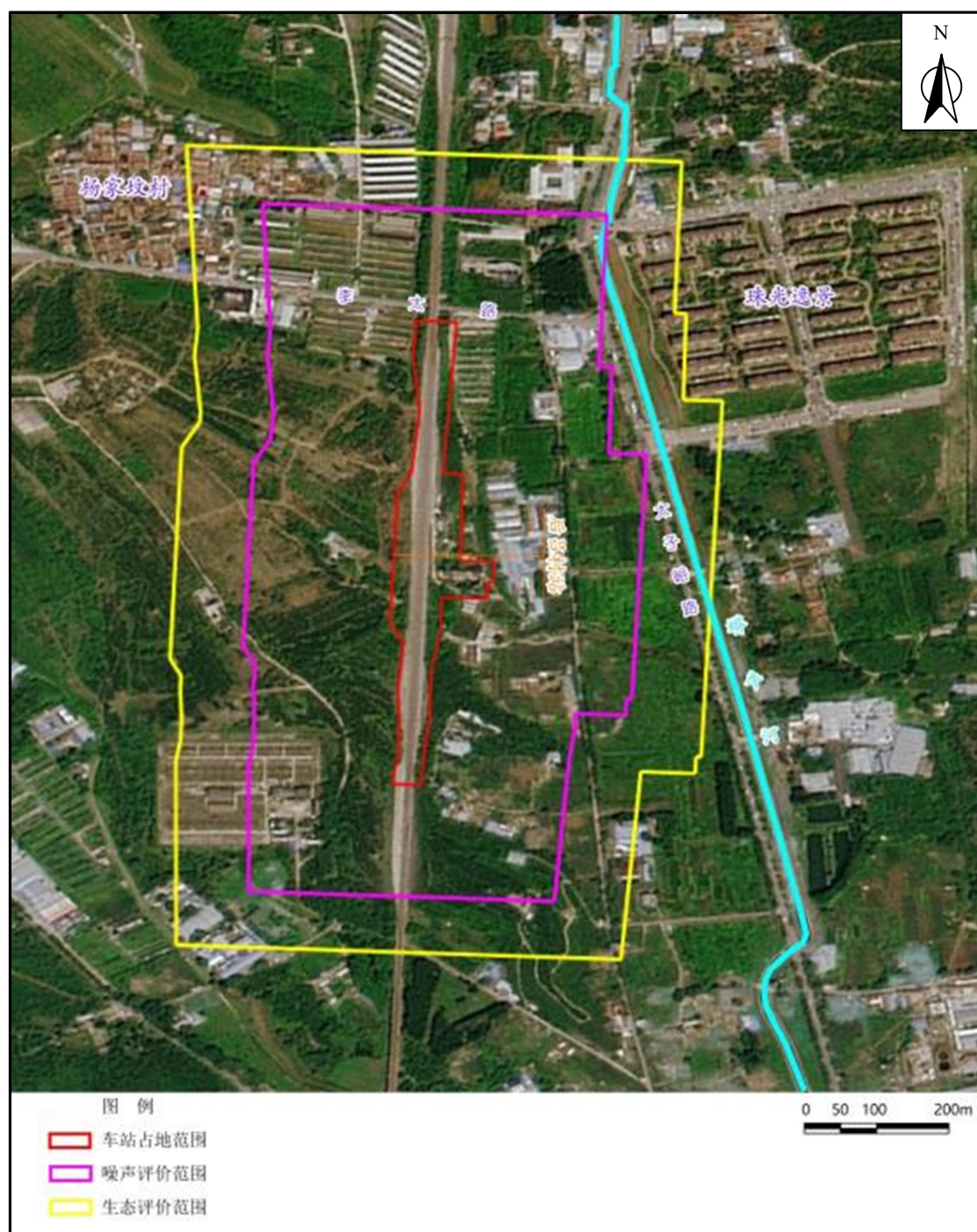
图 1.4-2 后吕村站评价范围图
