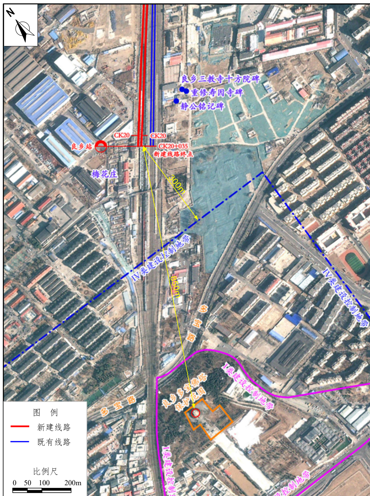
图 11.3-1 本工程与文物位置关系图
