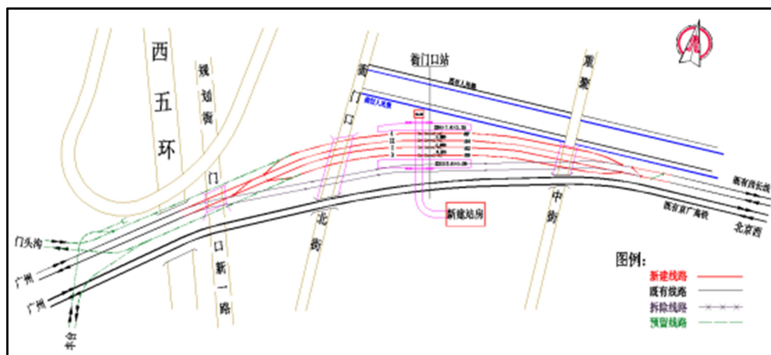
图 2.2-5 衙门口站示意图
