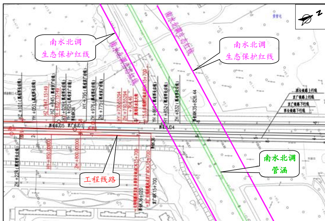
图 14.2-2 工程线路与南水北调生态保护红线位置关系
