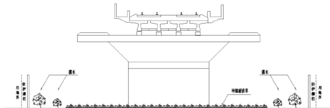
图 2.2-12 桥下绿化断面示意图
