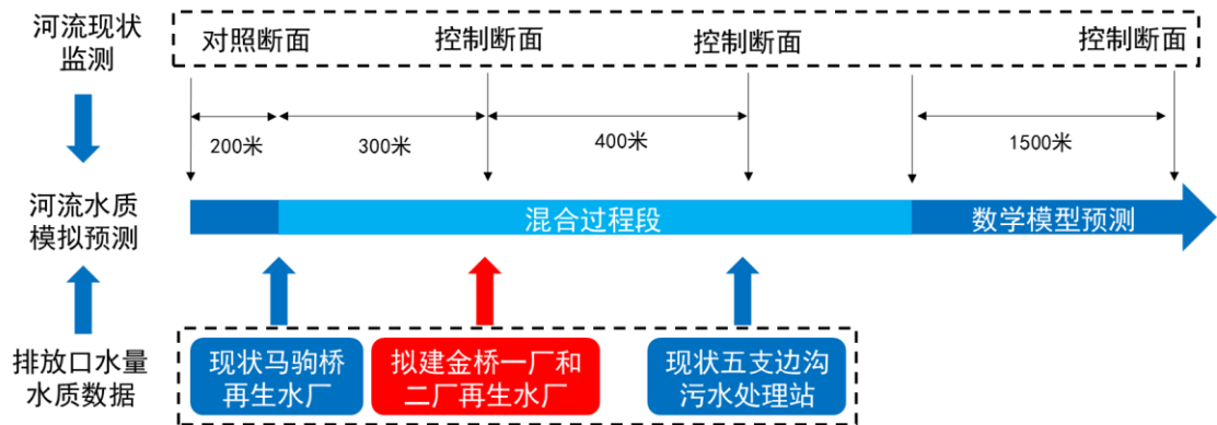
图 6-2 模型预测概化示意图
