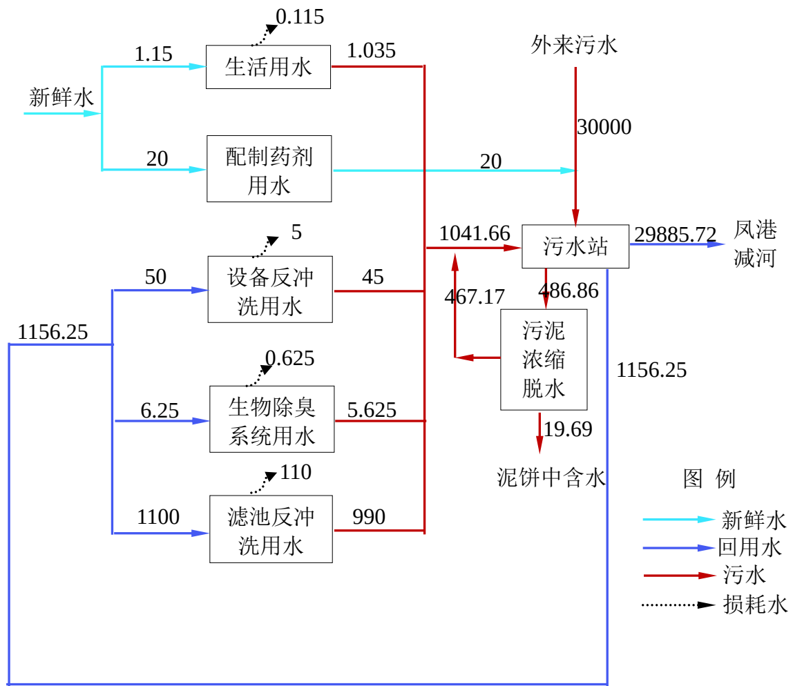
图 4-3 本项目非绿化季水平衡示意图 单位 t/d
