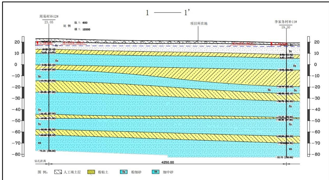
图 5-4 水文地质剖面图
