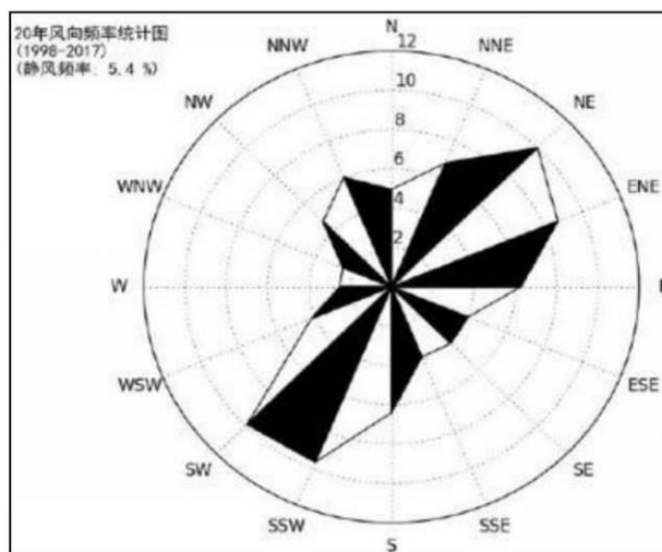
图 5-1 北京气象站 20 年风向玫瑰示意图
