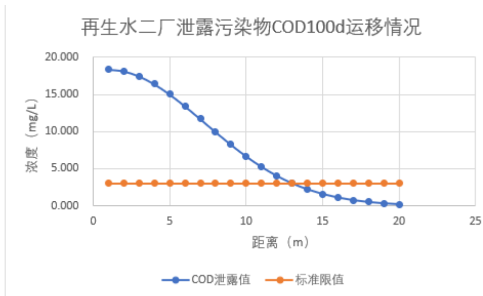
图 6-5 泄露污染物 COD100d 运移情况
