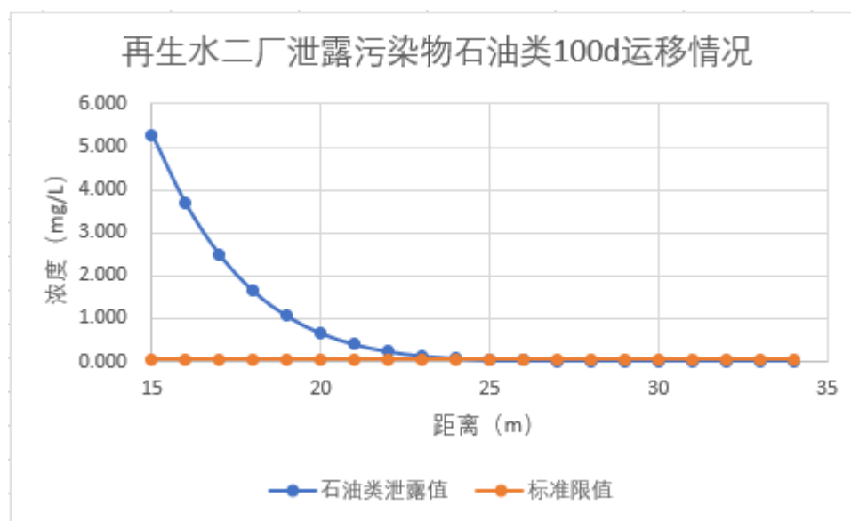
图 6-25 泄露污染物石油类 100d 运移情况
