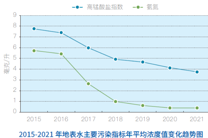
图 5-6 2015-2021 年地表水主要污染指标年平均浓度值变化趋势图
