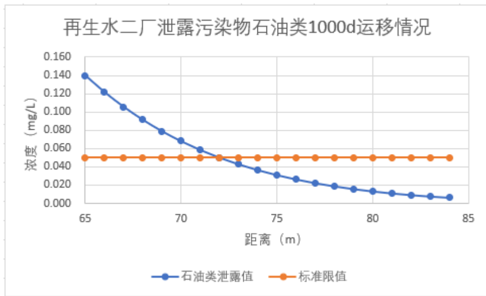
图 6-28 泄露污染物石油类 1000d 运移情况
