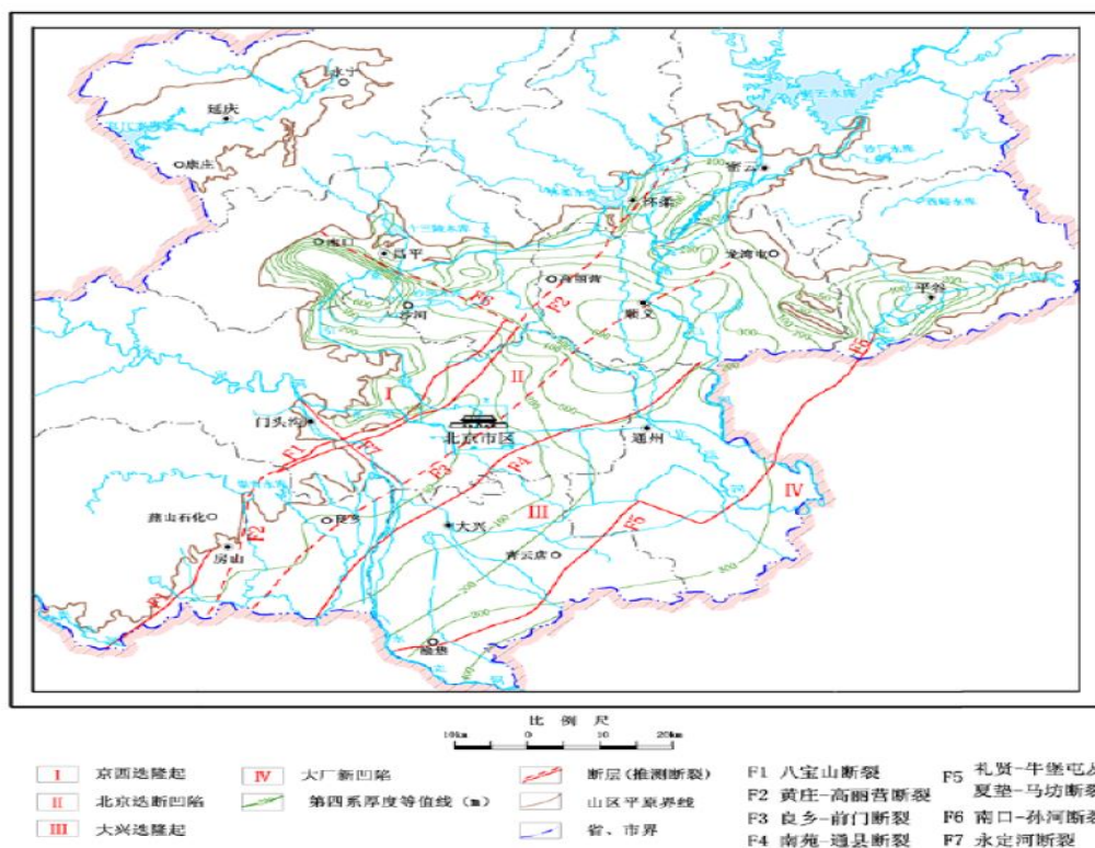
图 5-5 区域构造地质图
