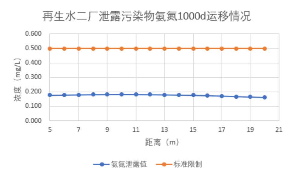
图 6-13 泄露污染物氨氮 1000d 运移情况
