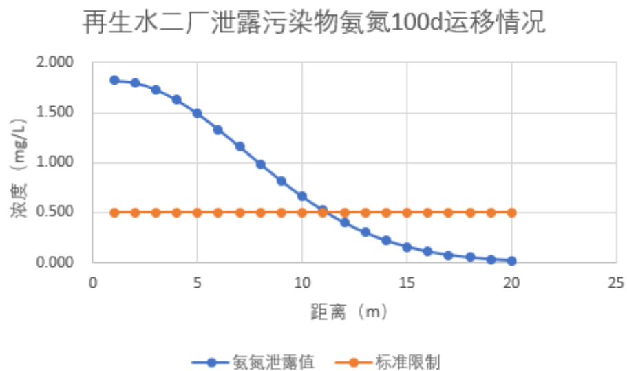
图 6-10 泄露污染物氨氮 100d 运移情况
