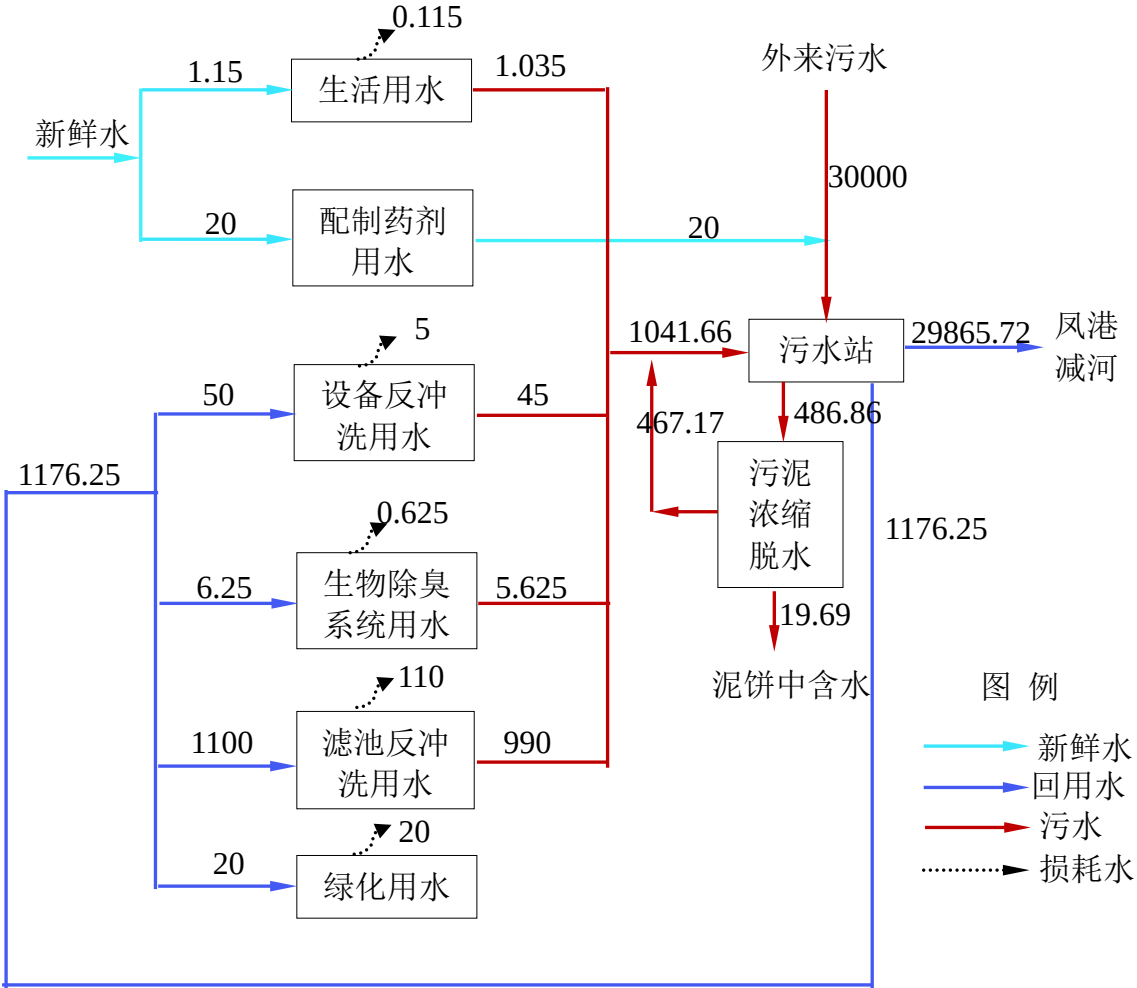
图 4-2 本项目绿化季水平衡示意图 单位 t/d
