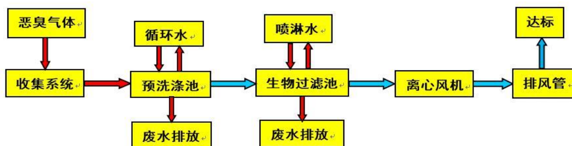
图 3-4 除臭工艺流程示意图
