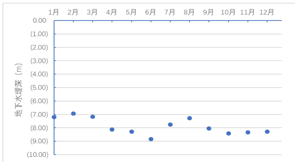
图 5-8 2022 年全年通州区马村自动监测站地下水埋深变化图
