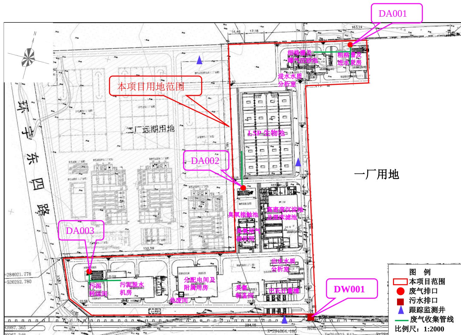
图 3-5 平面布置示意图
