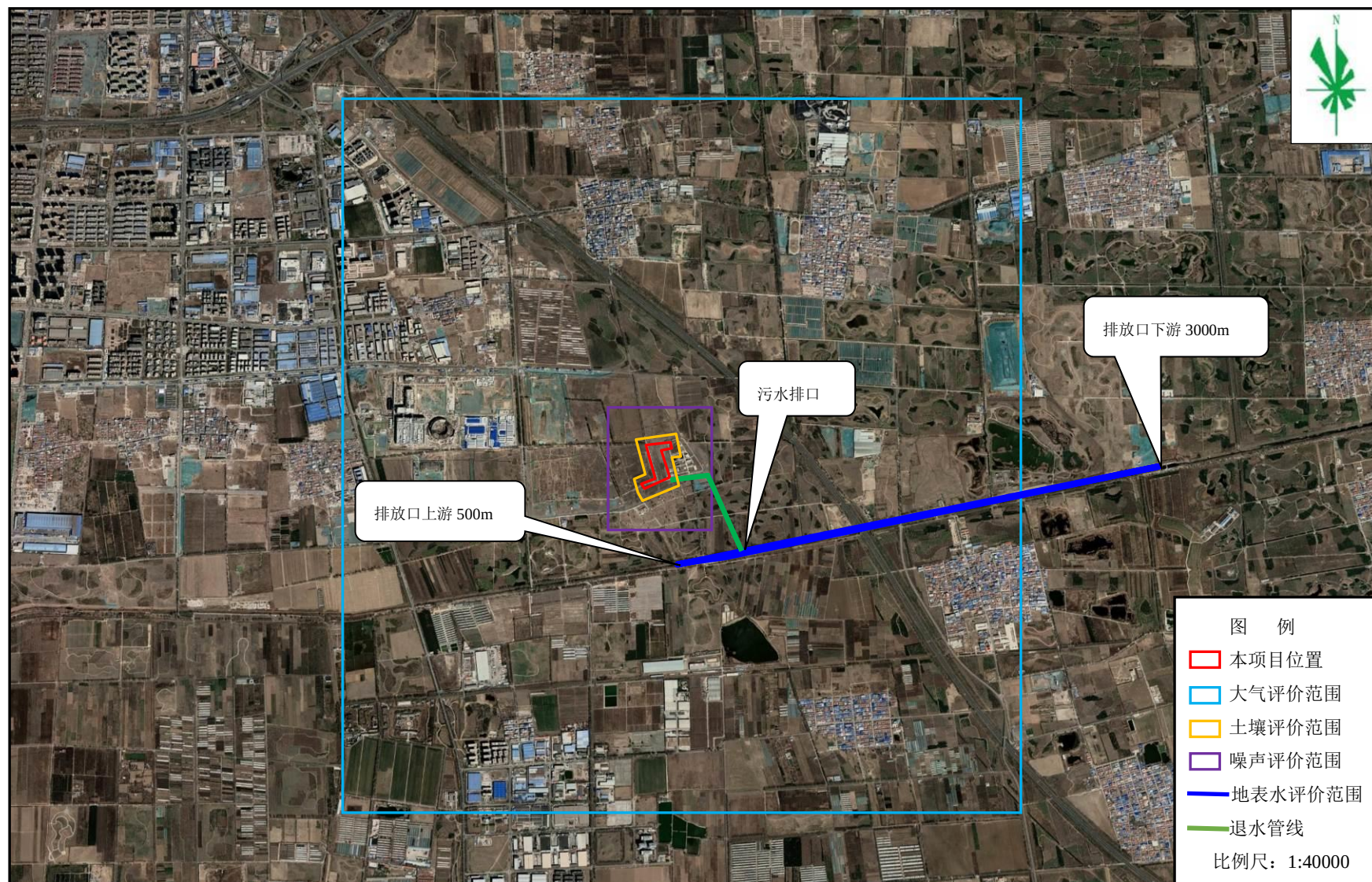
图 2-3 大气、土壤、噪声、地表水评价范围示意图
