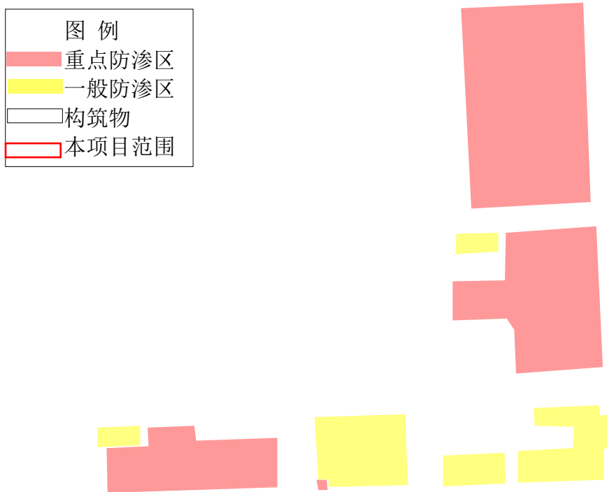
图 7.2-2 全厂分区防渗示意图
