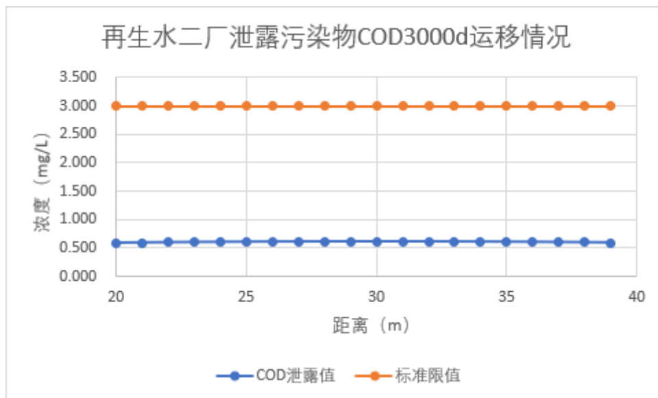
图 6-9 泄露污染物 COD3000d 运移情况
