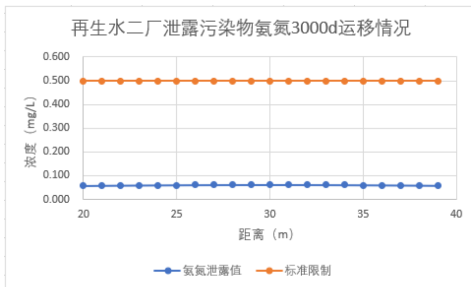
图 6-14 泄露污染物氨氮 3000d 运移情况
