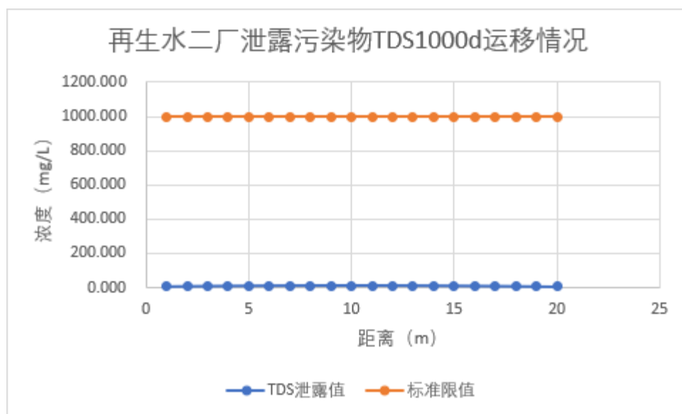
图 6-18 泄露污染物 TDS1000d 运移情况
