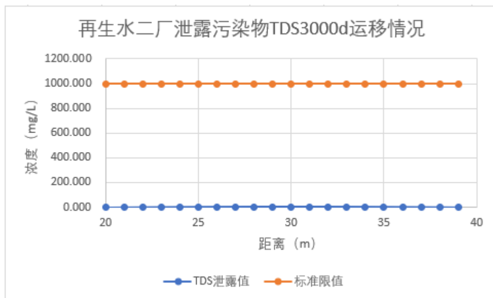
图 6-19 泄露污染物 TDS3000d 运移情况
