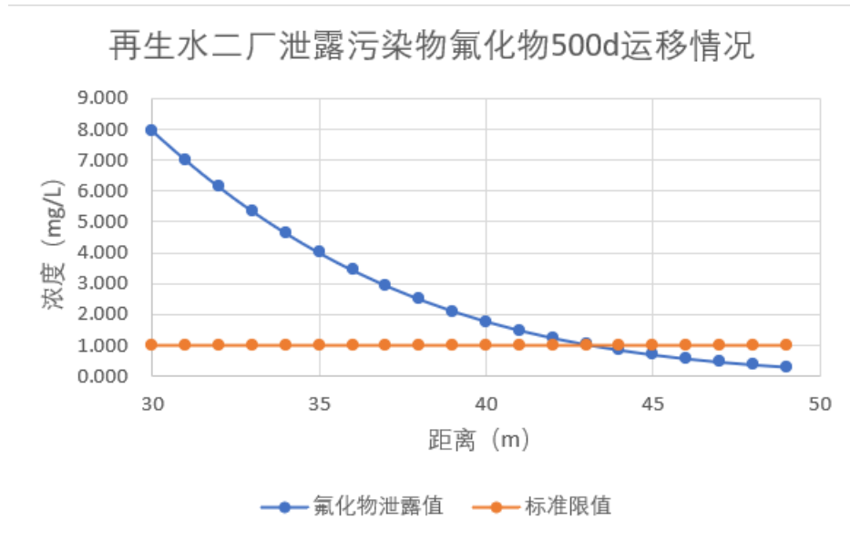
图 6-22 泄露污染物氟化物 500d 运移情况
