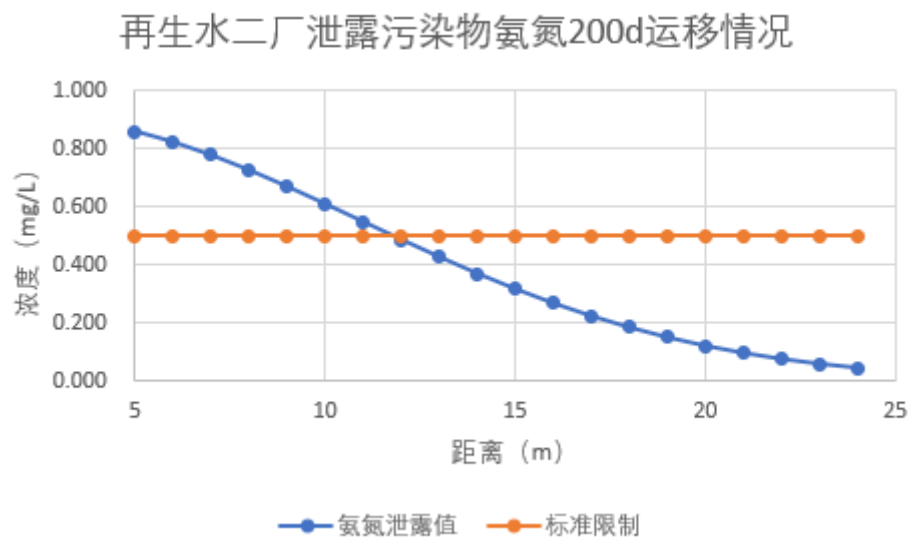
图 6-11 泄露污染物氨氮 200d 运移情况
