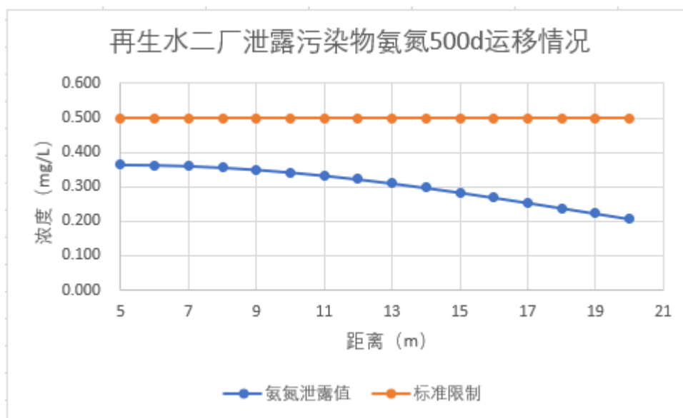
图 6-12 泄露污染物氨氮 500d 运移情况
