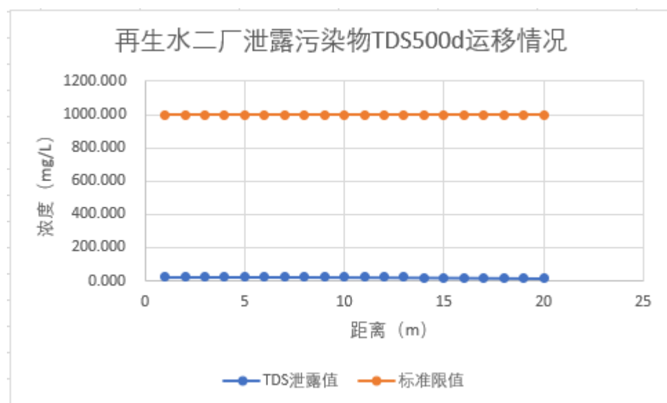
图 6-17 泄露污染物 TDS500d 运移情况
