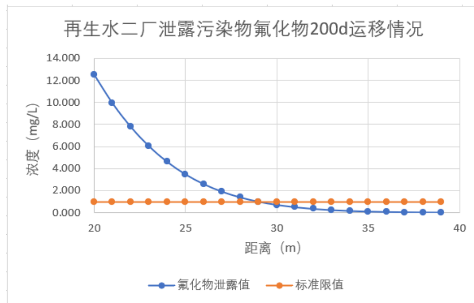
图 6-21 泄露污染物氟化物 200d 运移情况
