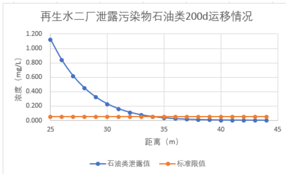
图 6-26 泄露污染物石油类 200d 运移情况
