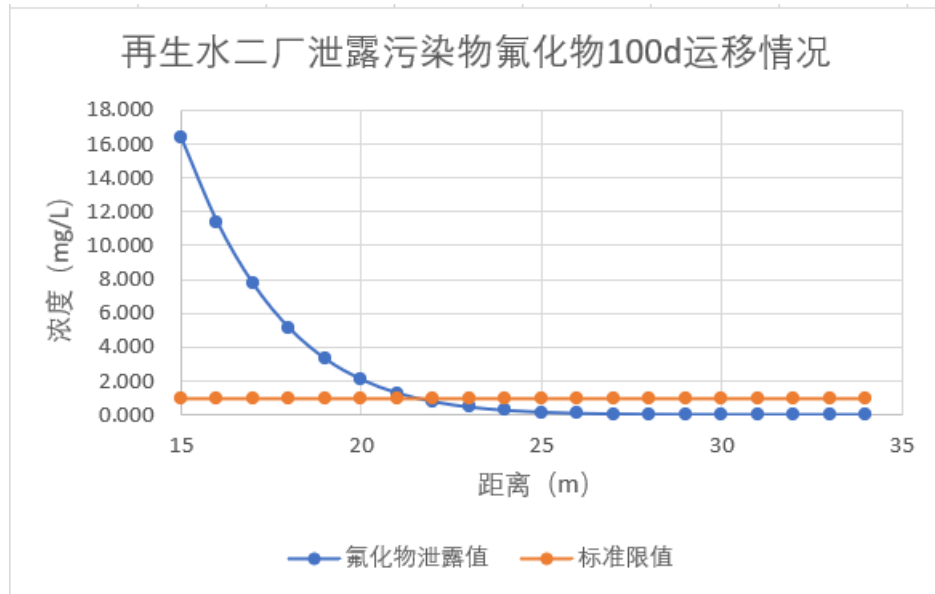
图 6-20 泄露污染物氟化物 100d 运移情况
