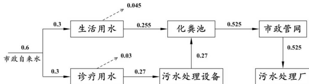
图3 水平衡图 单位：m 3 /d
