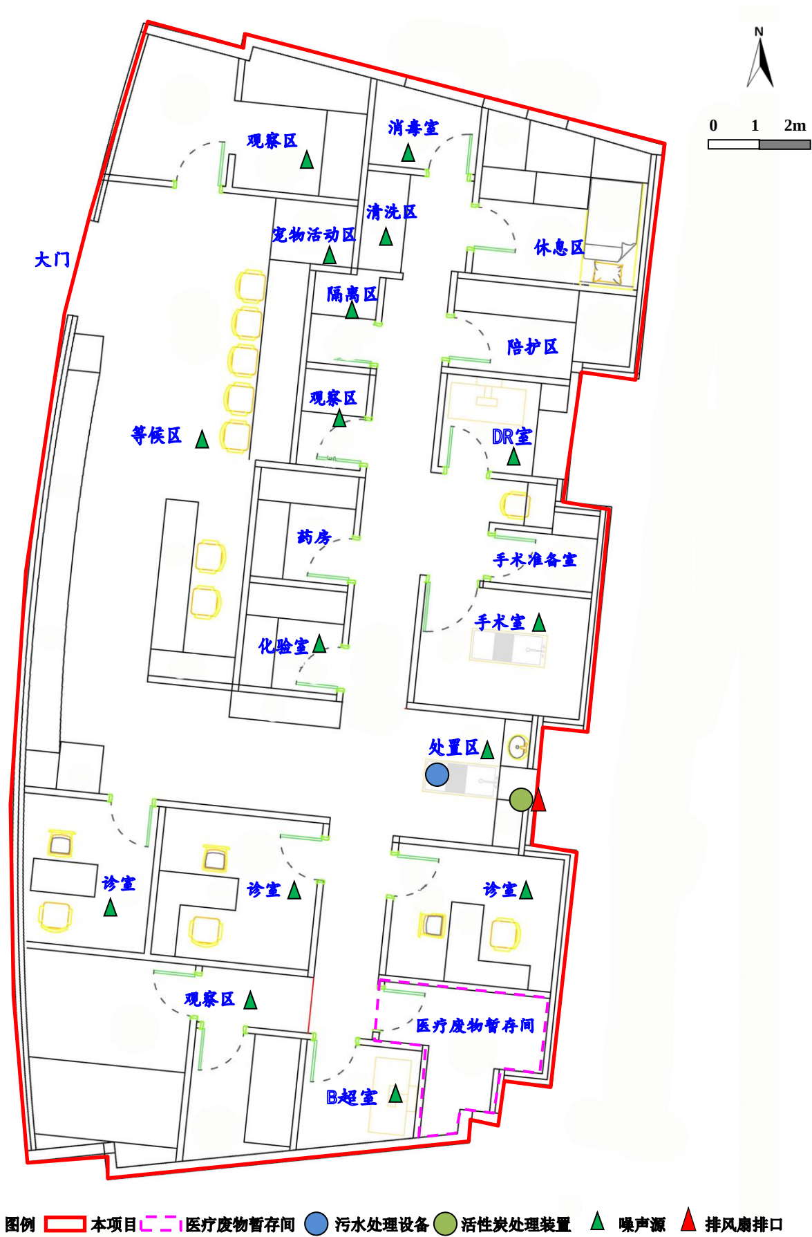
附图3 项目平面布局及污染源分布图
