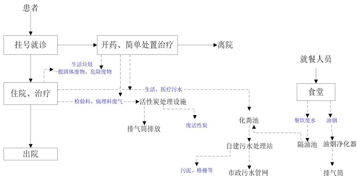
图 3.3-1 项目工艺流程及产排污节点
