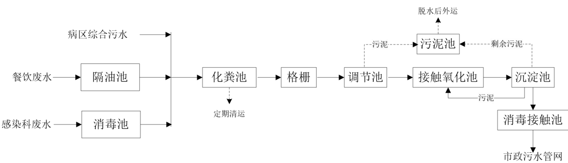
图 5.2-2 本项目污水处理工艺流程图
