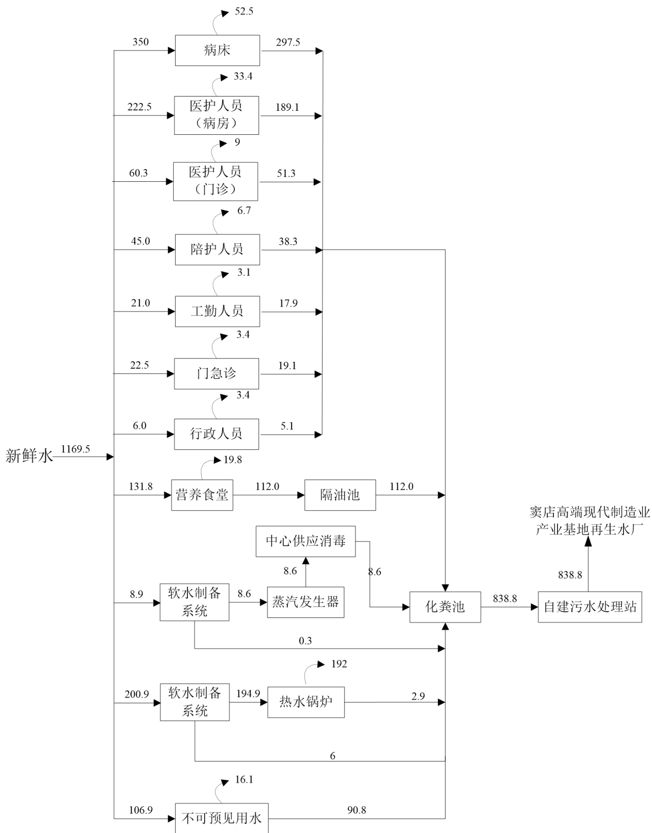
图 3.3-3 本项目水平衡图（非采暖季）
