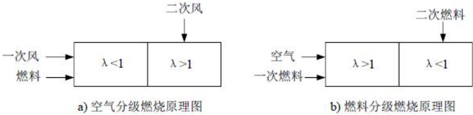
图 6.1-1 空气分级和燃料分级燃烧原理图
