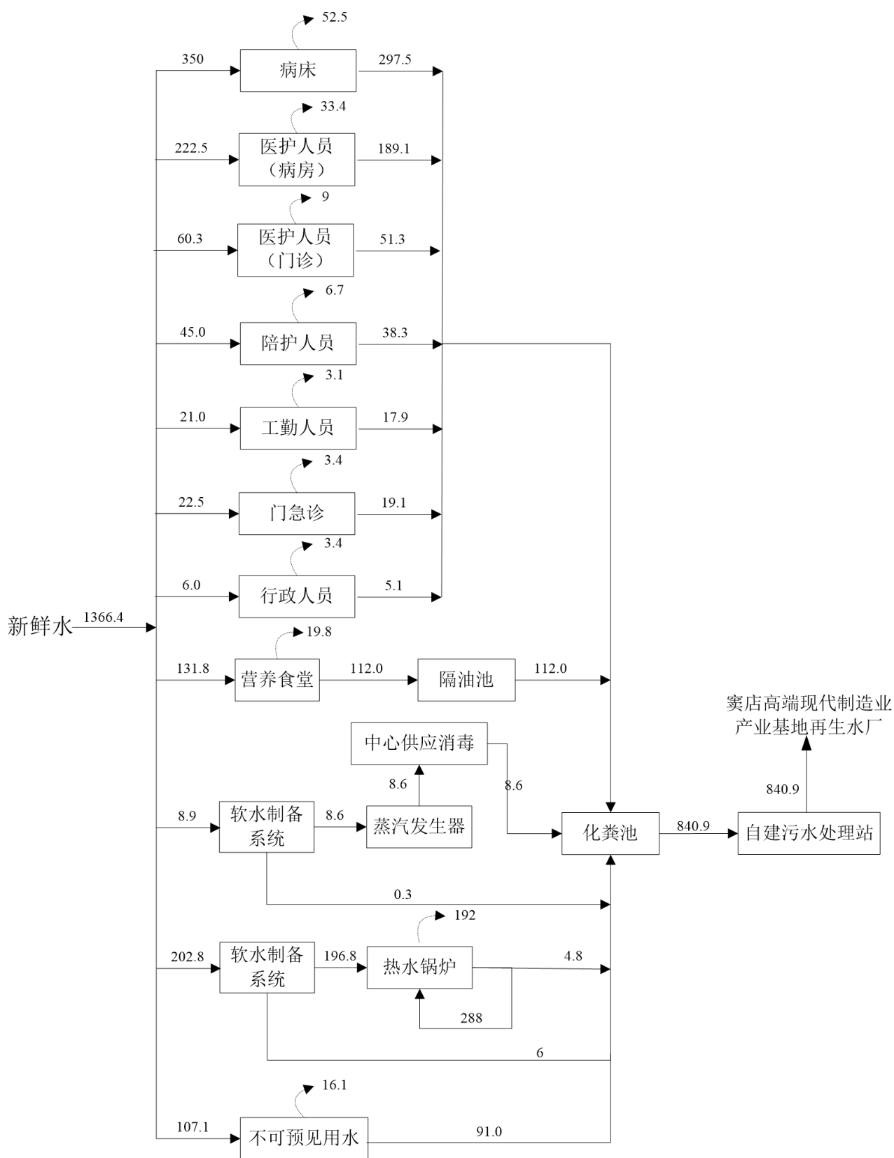
图 3.3-2 本项目水平衡图（采暖季）
